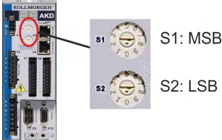
将 S1 设置为 8，将 S2 设置为 9
