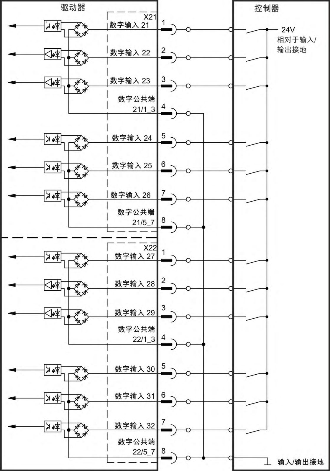
数字输入接线图 例如，漏类型连接
