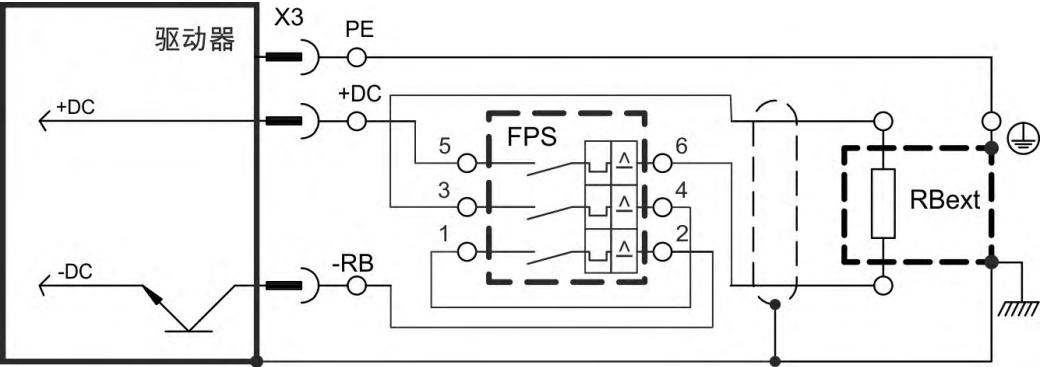
FPS:Fritzlen 直流电源开关
