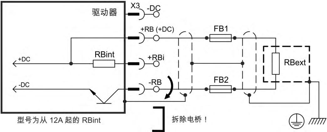
FB1 / FB2 保险功能
