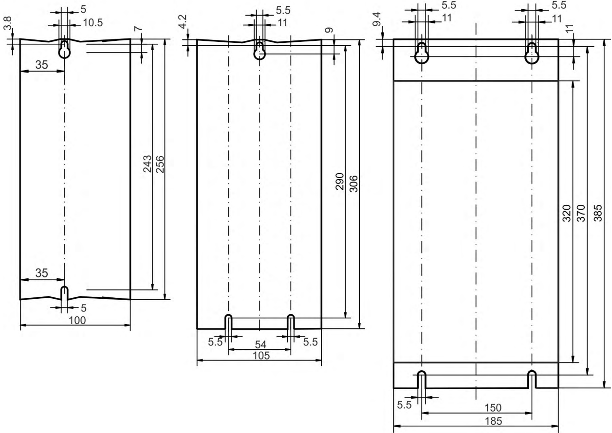
AKD 加长宽度 480V, 3A 至 12A
