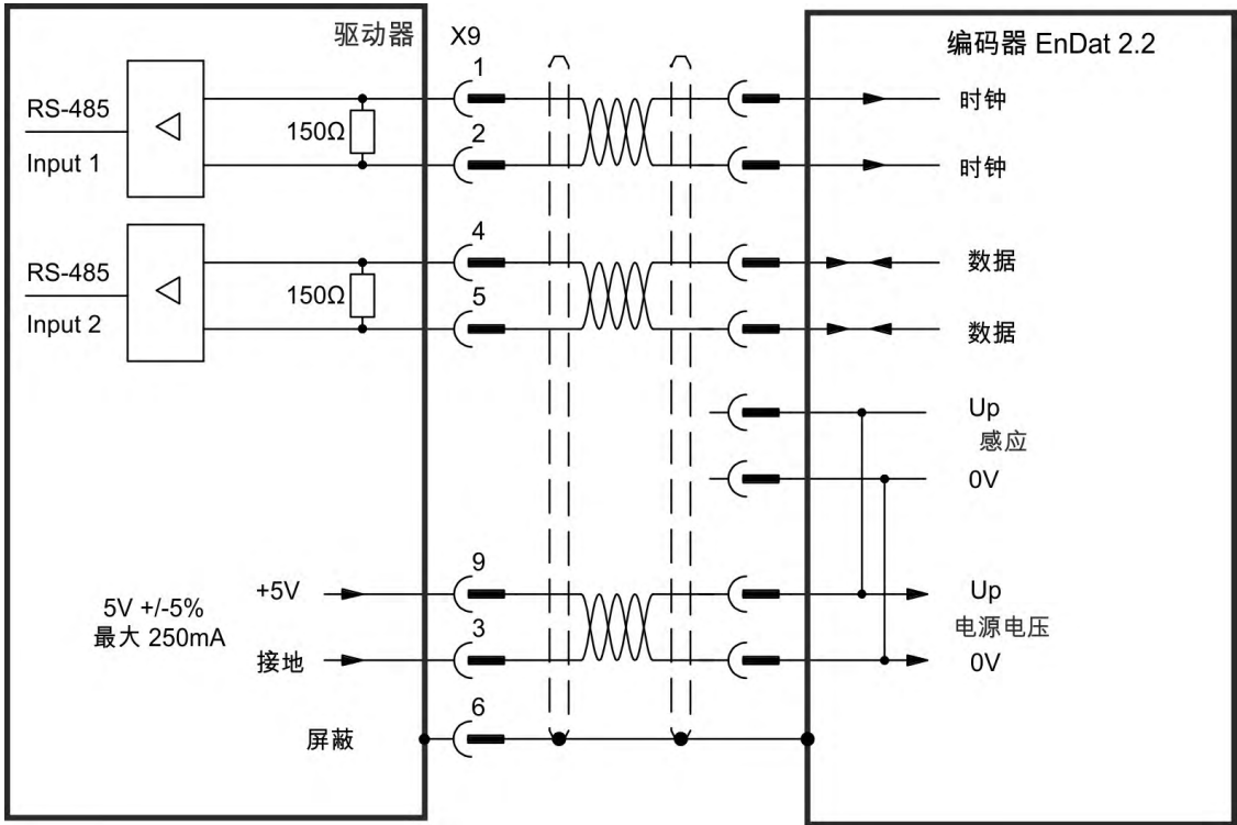
连接图
