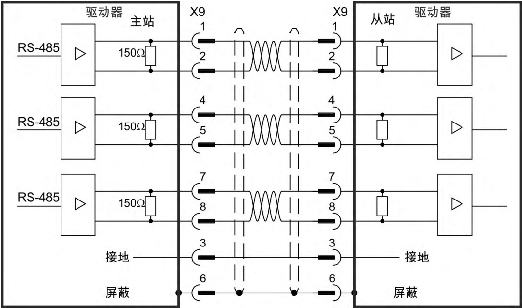
主从连接图，5V 信号等级 (X9) 的示例
